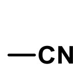
氰基
