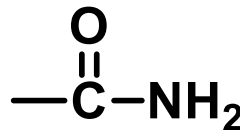
氨基甲酰基
